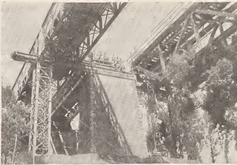
Aspecto do pilar de alvenaria do lado do Luso que foi consolidado
