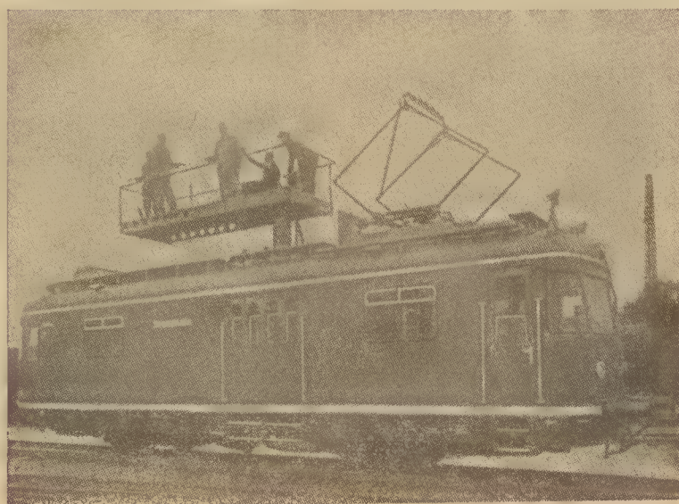
Veículo utilizado nas linhas férreas alemãs para inspeção e reparação das catenárias
