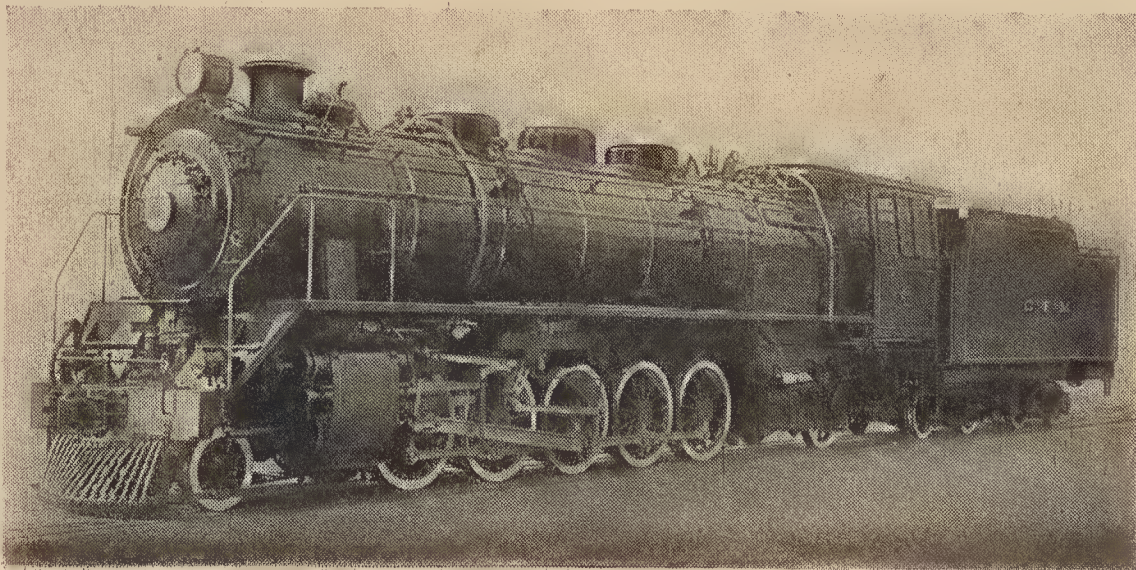
Locomotiva HENSCHEL, «tipo Santa Fé»
